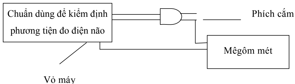
Hình 1: Sơ đồ kiểm tra điện trở cách điện
